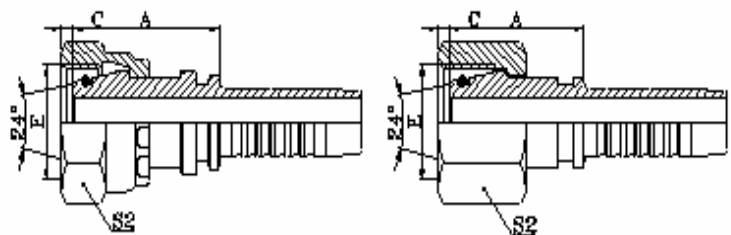
公制内螺纹 24°锥带 O 形圈轻系列 ISO 2151-2-DIN 3865 METRIC FEMALE 24° CONE O-RING L.T.
